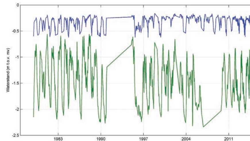
Figuur 14: Tijd-stijghoogtegrafiek van peilbuizen B22D0353 in blauw (filter boven slecht doorlatende laag, SDL) en B22D0354 in groen (filter in zandondergrond, onder SDL). Gegevens tussen 1992 en 1995 en tussen 2006 en 2010 (alleen B22D0354) ontbreken.
