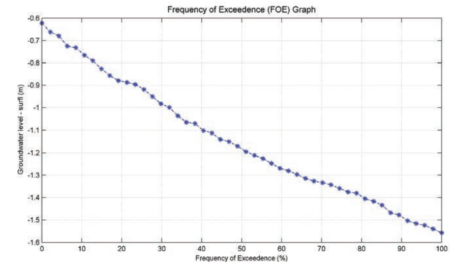
Figuur 6: Duurlijn van peilbuis B22D0359 (gemiddeld over 1978 tot en met 1990).
