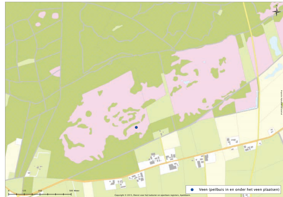
Figuur 27: Op deze locatie in het veen wordt aanbevolen om een peilbuis te plaatsen.
