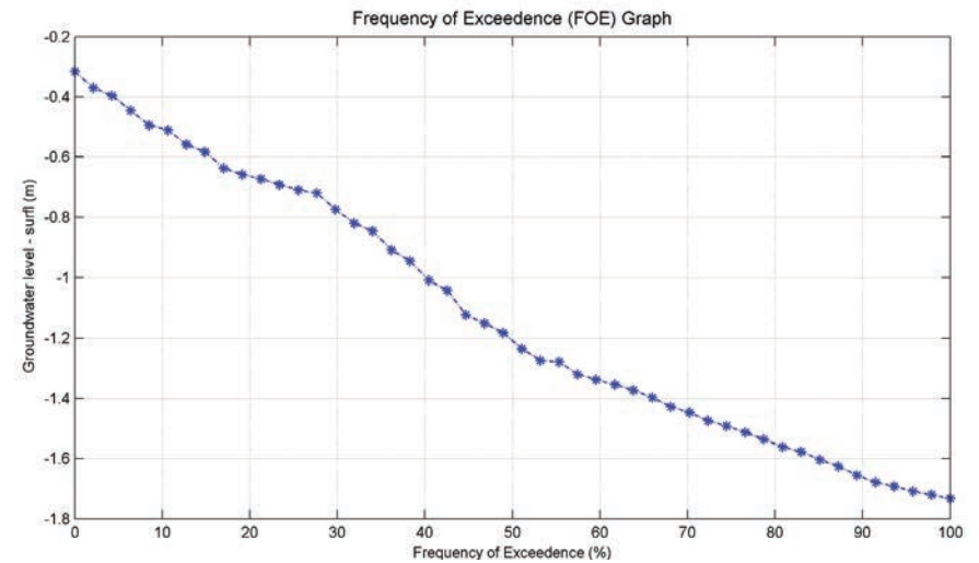
Figuur 4: Duurlijn van peilbuis B22D0357 (gemiddeld over 1978 tot en met 1990).
