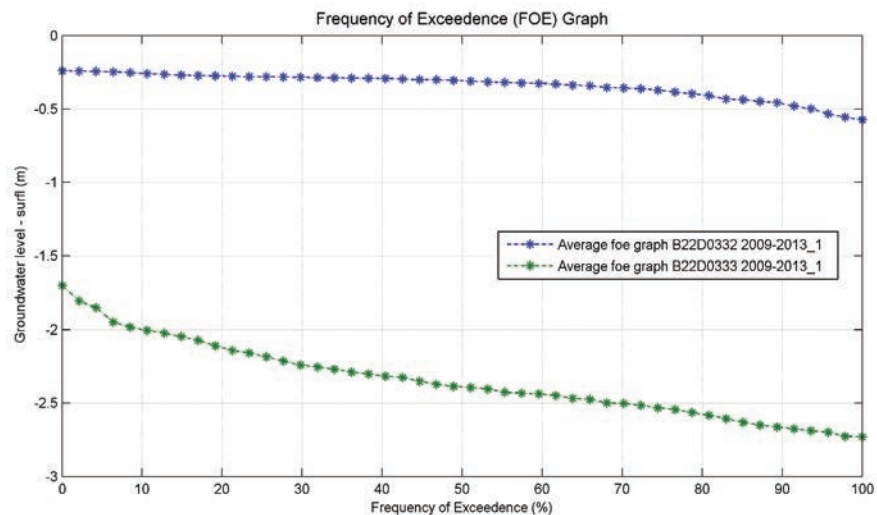
Figuur 13: Duurlijnen van peilbuizen B22D0332 (in de schijngrondwaterspiegel) en B22D0333 (in de zandondergrond) (gemiddeld over 2009 tot en met 2013).
