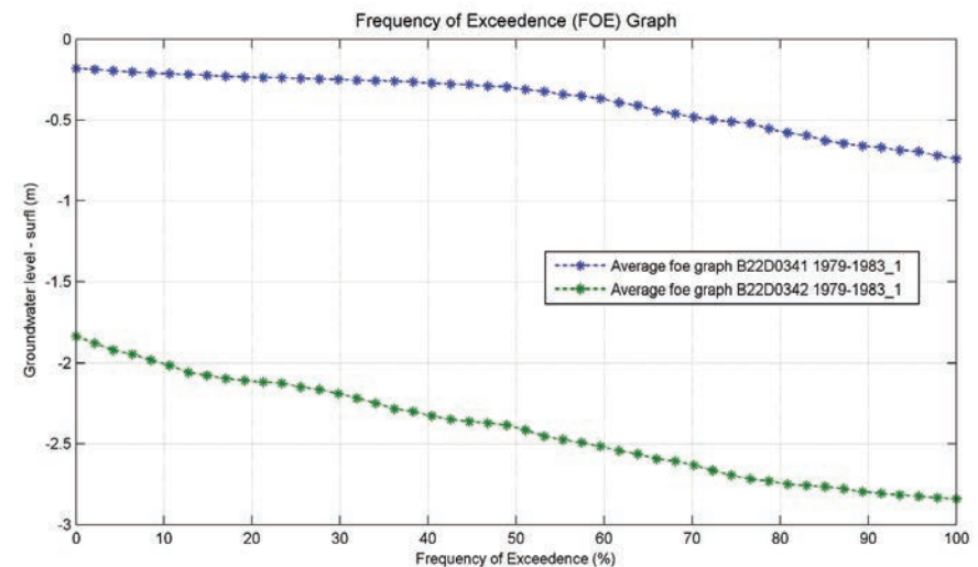
Figuur 15: Duurlijnen van peilbuizen B22D0341 (in de schijngrondwaterspiegel) en B22D0342 (in de zandondergrond) (gemiddeld over 1979 tot en met 1983).
