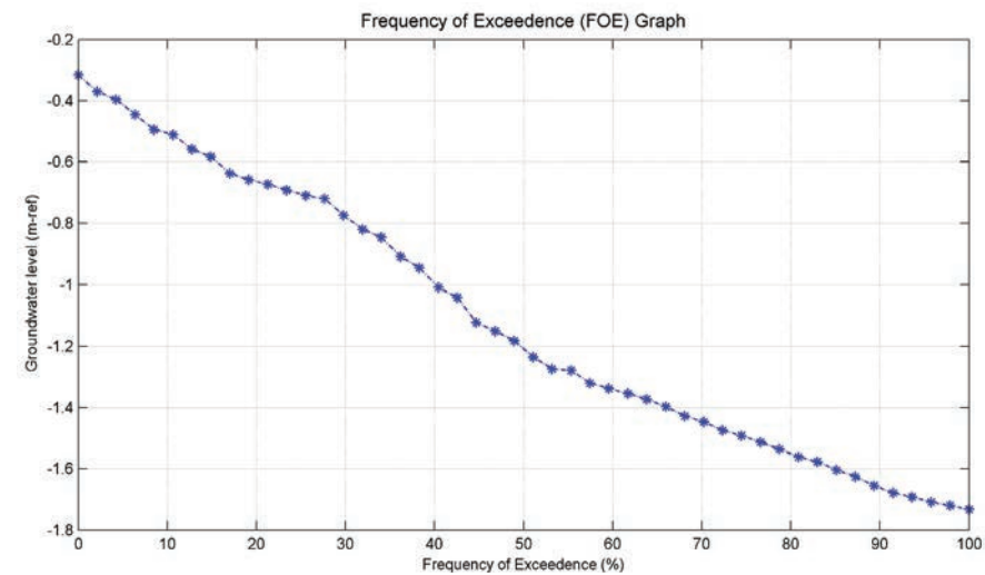
Figuur 5: Duurlijn van peilbuis B22D0358 (gemiddeld over 1978 tot en met 1990).
