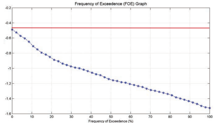
Figuur 9: Duurlijn van peilbuis B22D0616 (gemiddeld over 2004 tot en met 2014) met maaiveldhoogte (rode lijn) van de locatie met de Pioniervegetatie van snavelbiezen (H7150) ingetekend.
