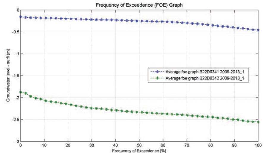
Figuur 14: Duurlijnen van peilbuizen B22D0341 (in de schijngrondwaterspiegel) en B22D0342 (in de zandondergrond) (gemiddeld over 2009 tot en met 2014).
