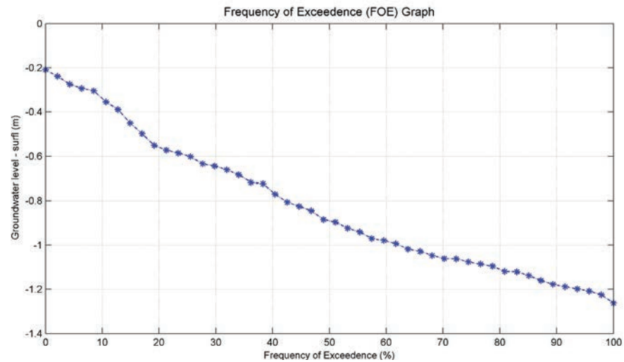
Figuur 3: Duurlijn van peilbuis B22D0339 (gemiddeld over 1978 tot en met 1990).
