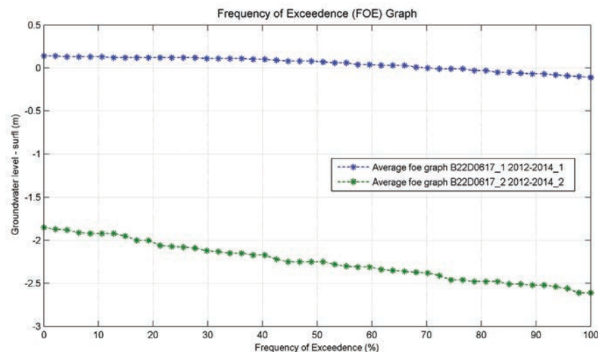
Figuur 11: Duurlijn van peilbuis B22D0617 (in de schijngrondwaterspiegel en de zandondergrond) (gemiddeld over 2012 tot en met 2014).
