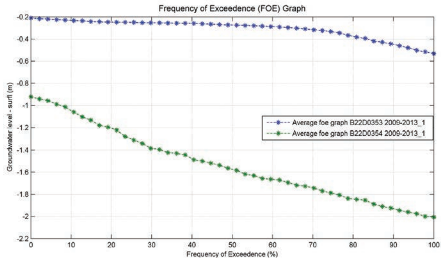
Figuur 12: Duurlijnen van peilbuizen B22D0353 (in de schijngrondwaterspiegel) en B22D0354 (in de zandondergrond) (gemiddeld over 2009 tot en met 2013).
