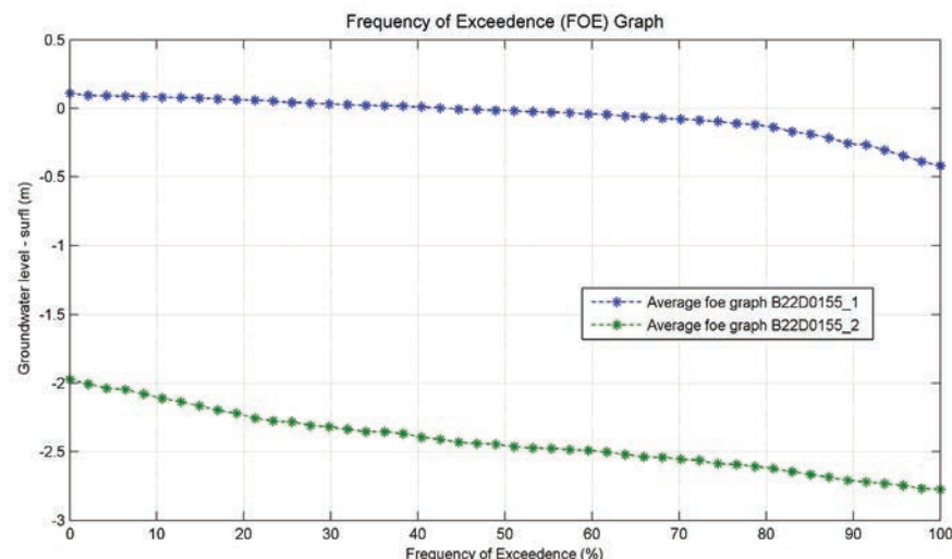
Figuur 10: Duurlijn van peilbuis B22D0155 (in de schijngrondwaterspiegel en de zandondergrond) (gemiddeld over 2009 tot en met 2013).
