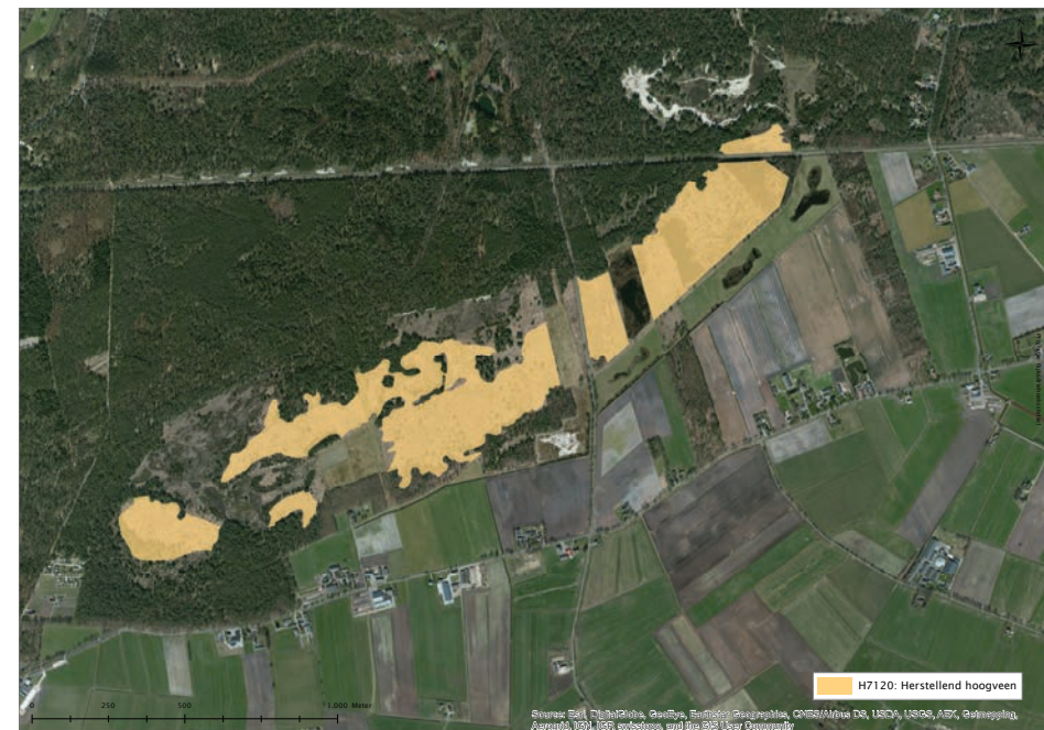
Figuur 7: Beerzerveld met in geel habitatype Herstellend hoogveen aangegeven (gebaseerd op de aangepaste habitattypenkaart, zie 3.5.2), dat ruwweg overeenkomt met de aanwezigheid van slecht doorlatende lagen.
