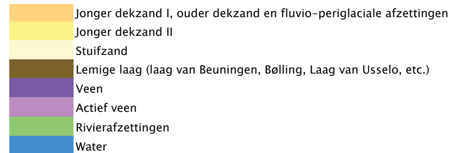
Figuur 5: Ontstaanswijze van het Beerzerveld. Door vernatting in het Holoceen trad er veenvorming op (II), daarna is het gebied overstoven (III) en zijn er veenputten gegraven (IV).
